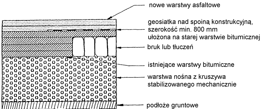
Rys. 5. Wzmocnienie nawierzchni asfaltowej w strefie poszerzenia nawierzchni
