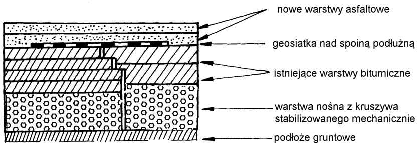
Rys. 5. Wzmocnienie nawierzchni asfaltowej w strefie poszerzenia nawierzchni
