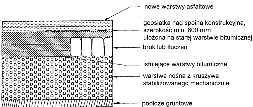
Rys. 5. Wzmocnienie nawierzchni asfaltowej w strefie poszerzenia nawierzchni
