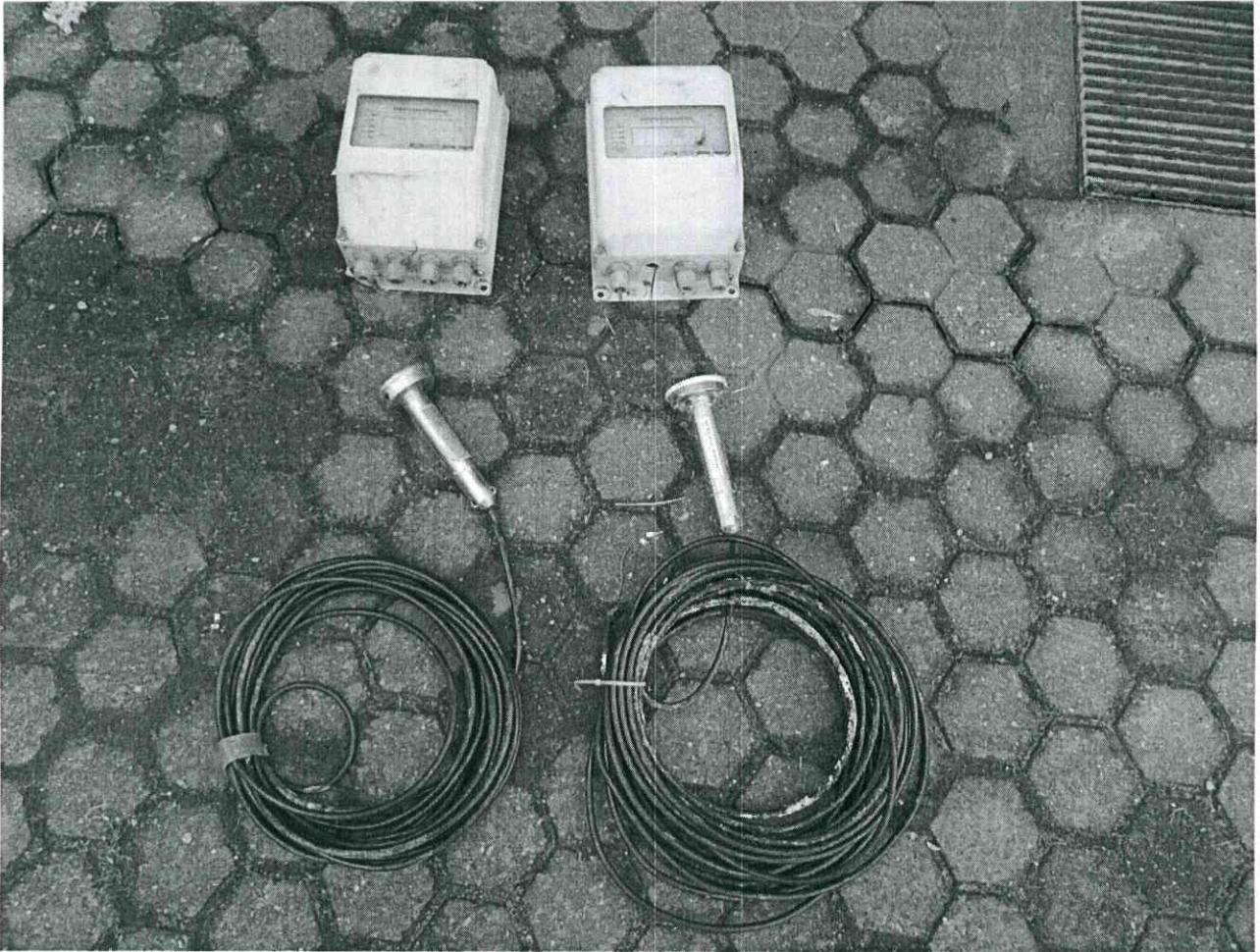
Sonda hydrostatyczna poziomu z miernikiem Oczyszczalnia ścieków Mleczno nr ew: 06 658 / 188
