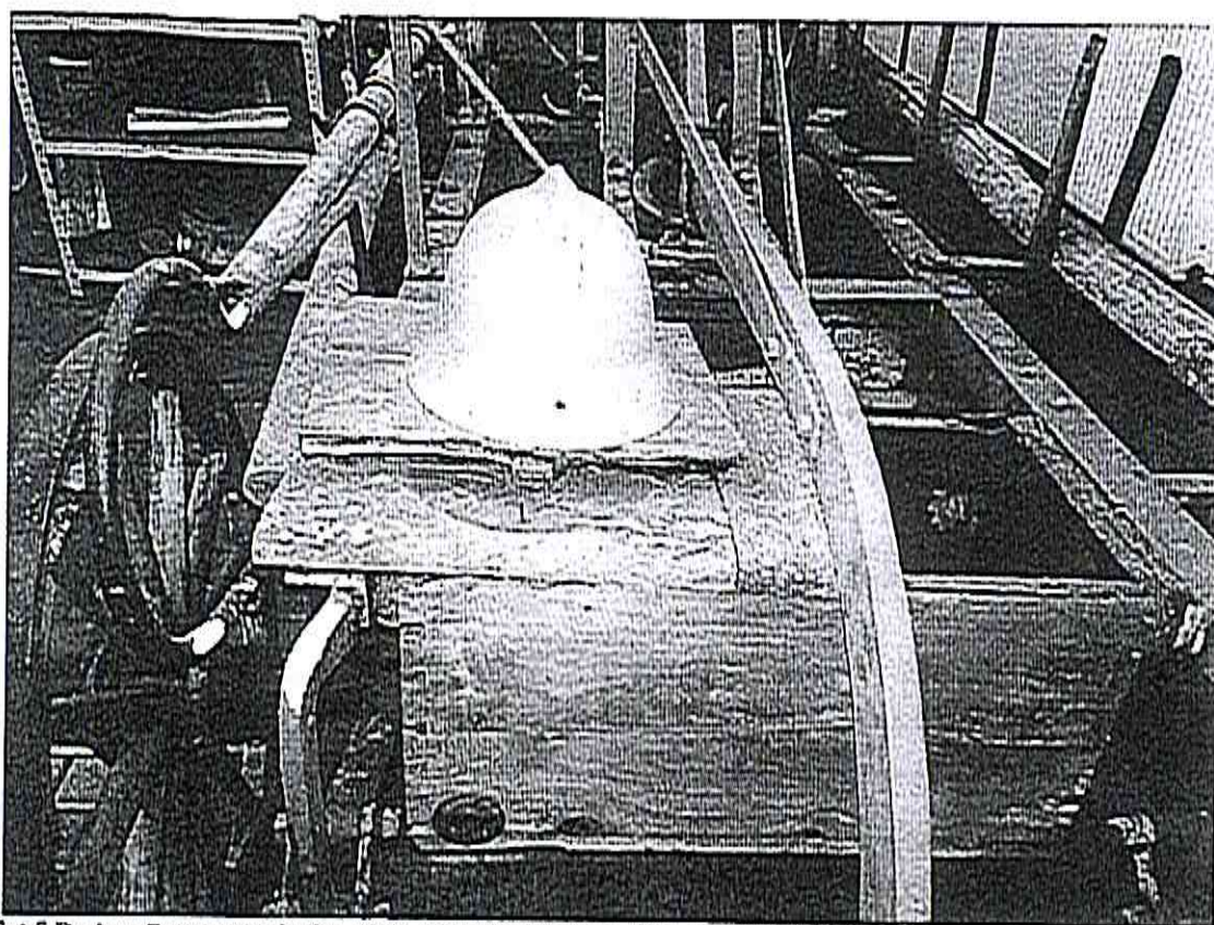
Fot 5 Rudna, Pompka strażacka, 1912. Fabryka Fladera. Stan na 2016. Widoczny zły stan wozu strażackiego z licznymi ubytkami, ogniskami korozji, zbutwiałym drewnem, przemalowaniami powierzchni. Helm strażacki również przemalowany.
