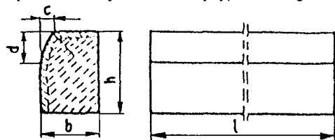
Rys. 2.1. Krawężnik betonowy typu ulicznego
